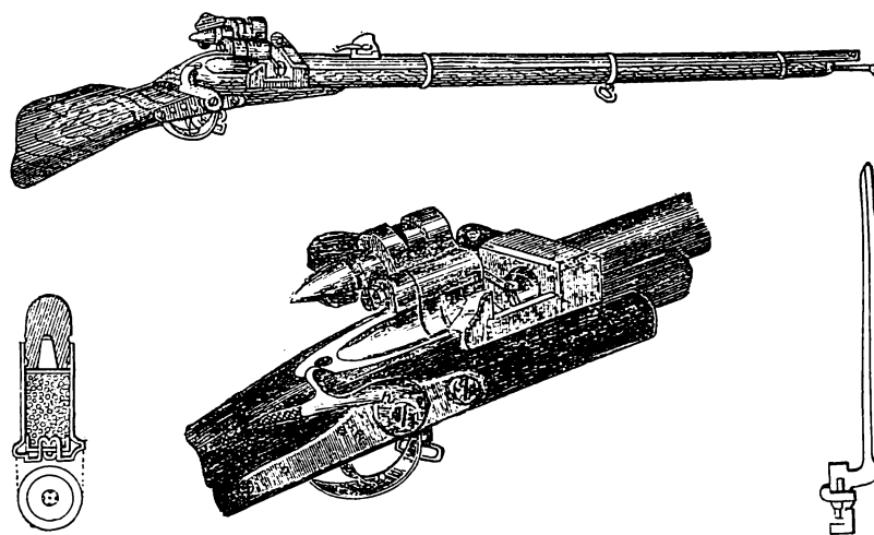
Ударная винтовка Крынка бывшая на вооруженіи Л.-Гв. Финляндскаго полка съ 1869 по 1875 годъ.
