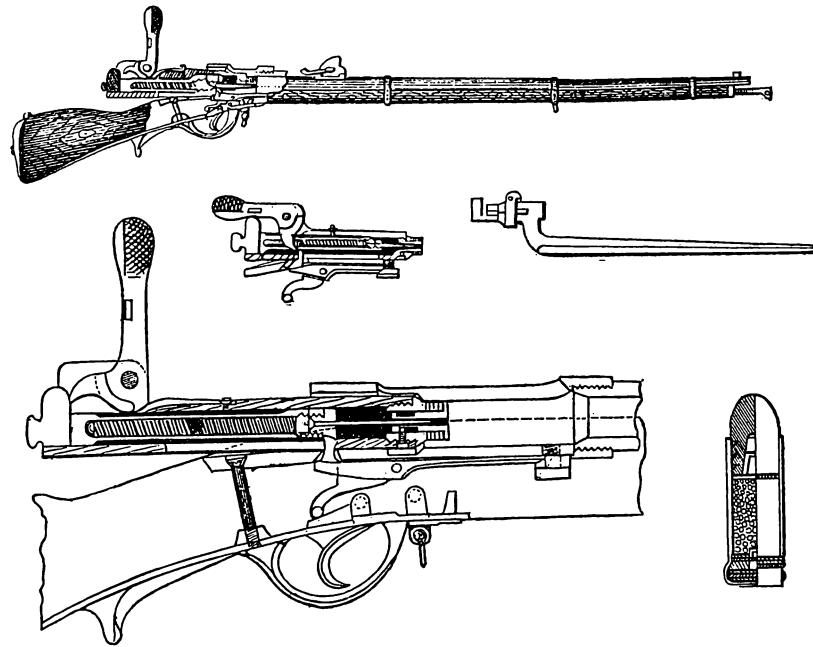
Игольчатая винтовка Карле бывшая на вооруженіи Л.-Гв. Финляндскаго полка съ 1868 по 1869 годъ.
