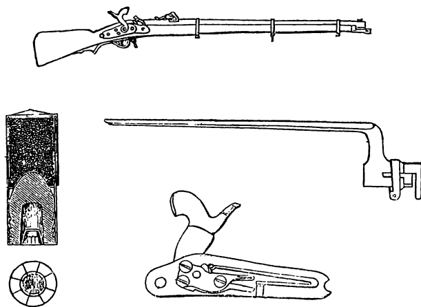
6-ти линейная винтовка бывшая на вооруженіи Л.-Гв. Финляндскаго полка съ 1860 по 1868 годъ.
